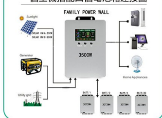
一個主機搭配四個電池箱連接圖
